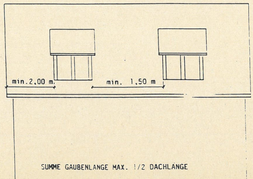
SCHLEPPGAUBEN
