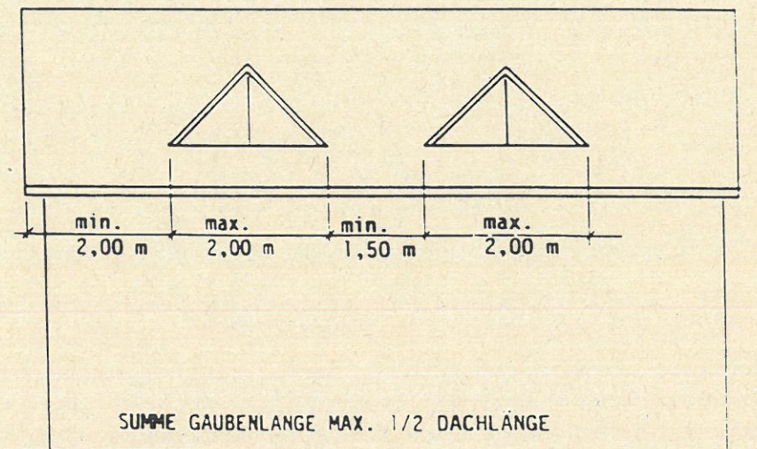
DREIECKSGAUBE
