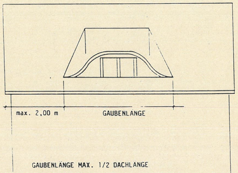
OCHSENAUGENGAUBE
