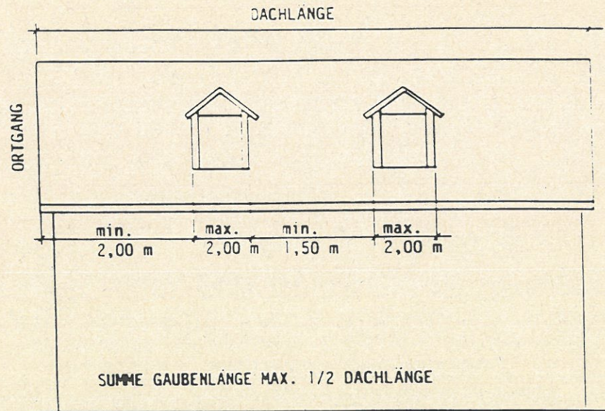
(giebelständige Gaube)
